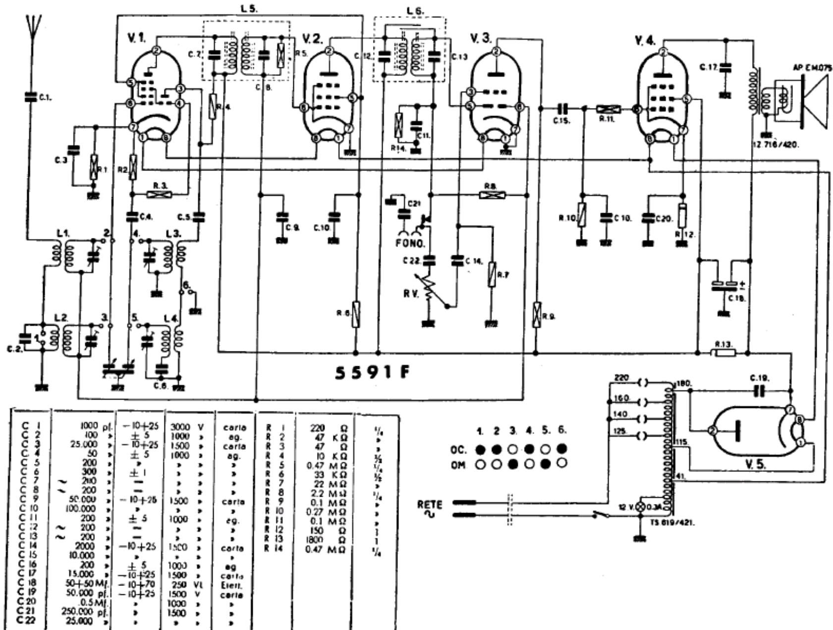
PHONOLA (S. A. FIMI) - Onde medie e onde corte da 18 a 52 metri. Media frequenza a 468 kc/s. Potenza d'uscita 2,3 watt.
